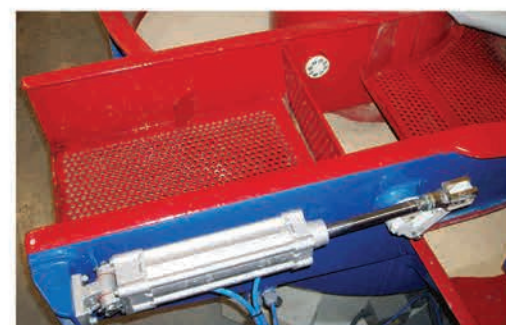
Pneumatische Separierung
